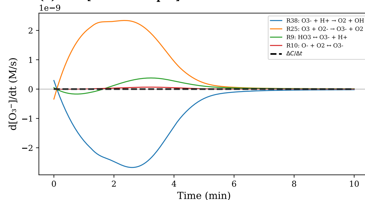
(d) O 3 - [final=0.00 pM]
